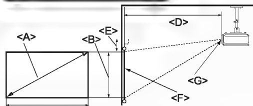
Installation au plafond
