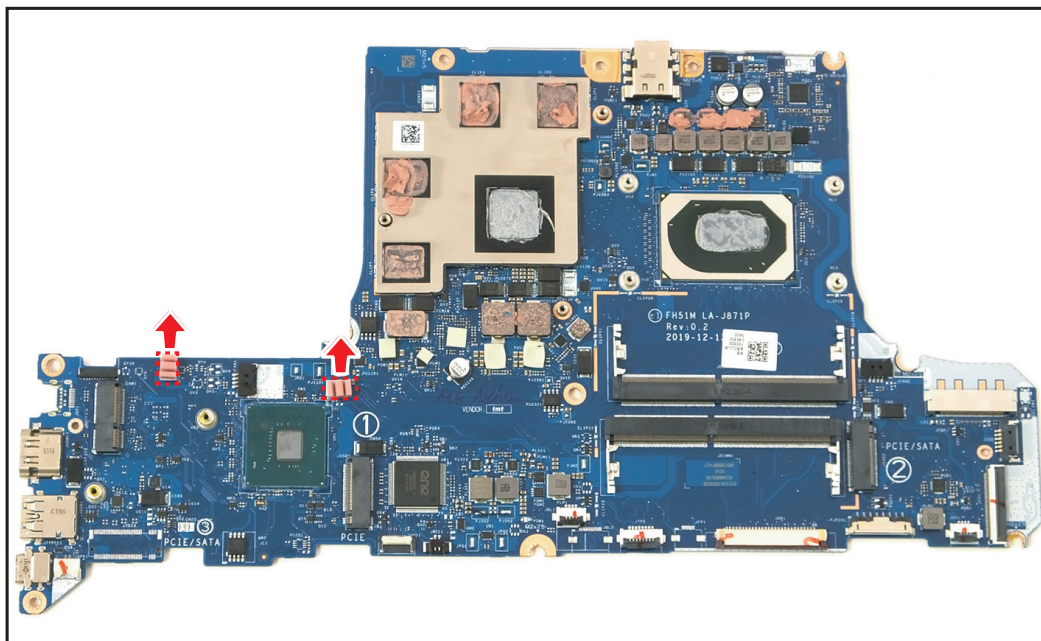
Figure 1-25. Retirer les guides en caoutchouc
