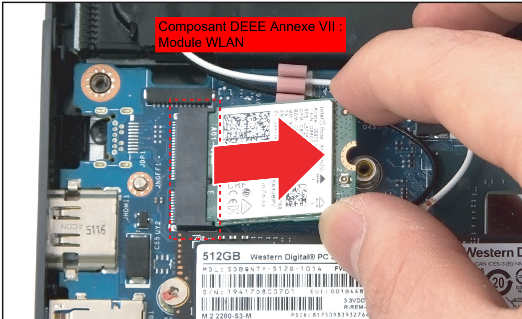
Figure 1-10. Retirer le module WLAN
