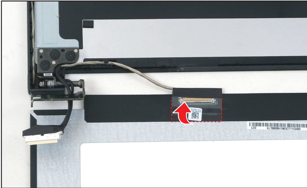
Figure 1-41. Détacher le Mylar
