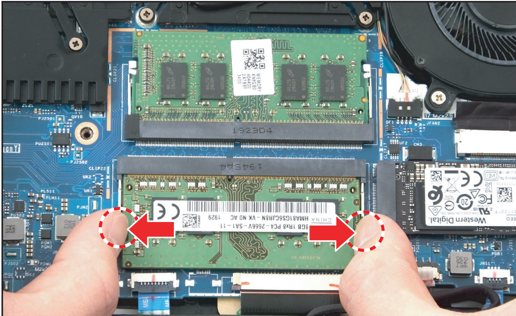
Figure 1-11. Détacher les clips du module
