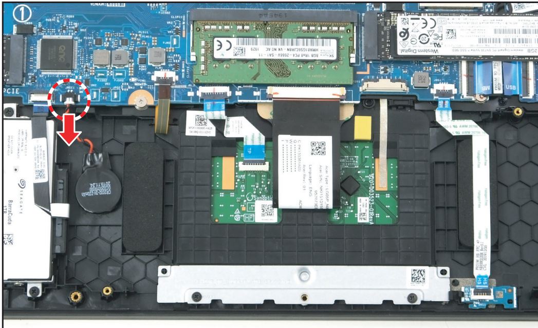
Figure 1-30. Débrancher le câble de la pile RTC
