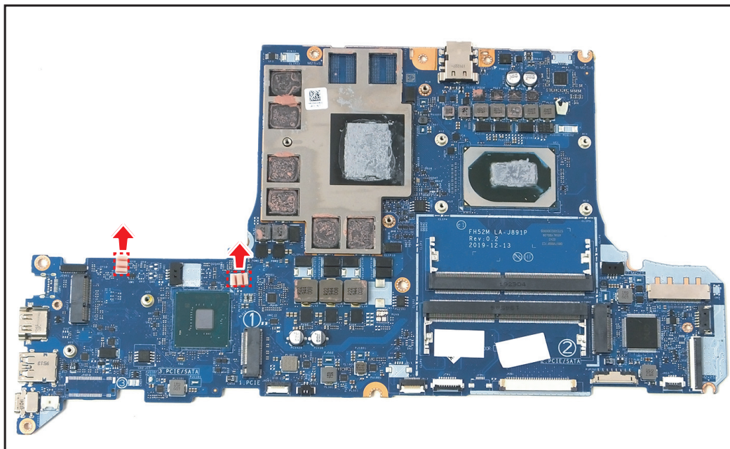
Figure 1-29. Retirer les guides en caoutchouc
