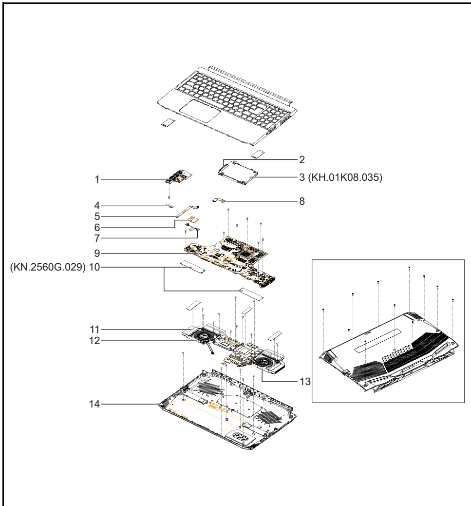
Figure 1-1. Vue éclatée de l'assemblage principal
