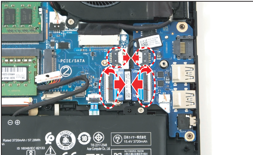
Figure 1-17. Débrancher les câbles
