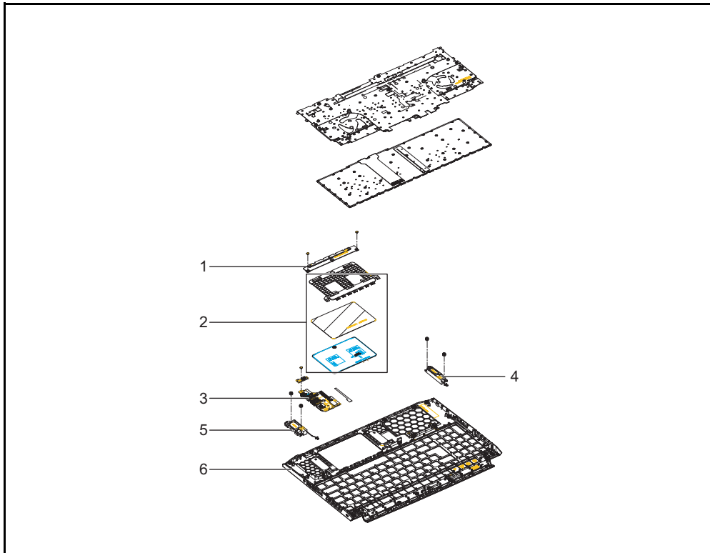
Figure 1-2. Vue éclatée de l'assemblage du boîtier supérieur
