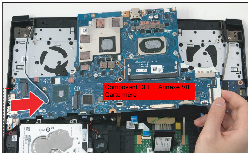
Figure 1-24. Retirer la carte mère
