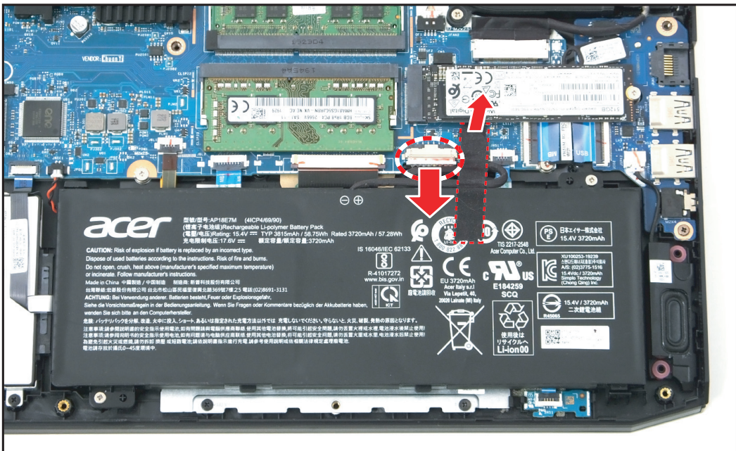
Figure 1-5. Débrancher le câble de la batterie
