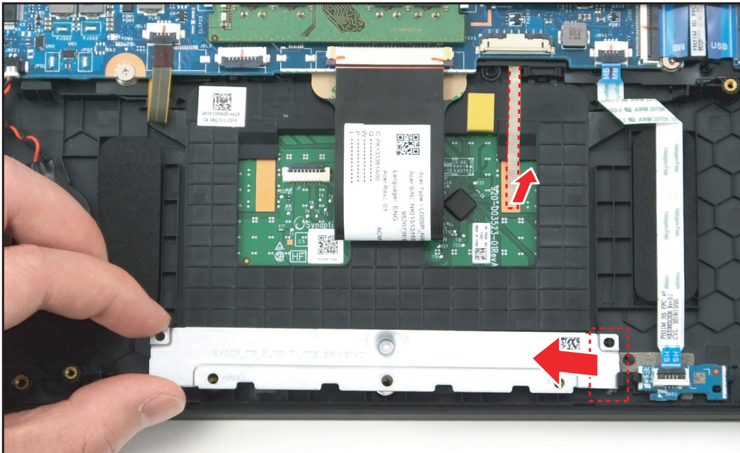
Figure 1-34. Retirer le support du socle du pavé tactile
