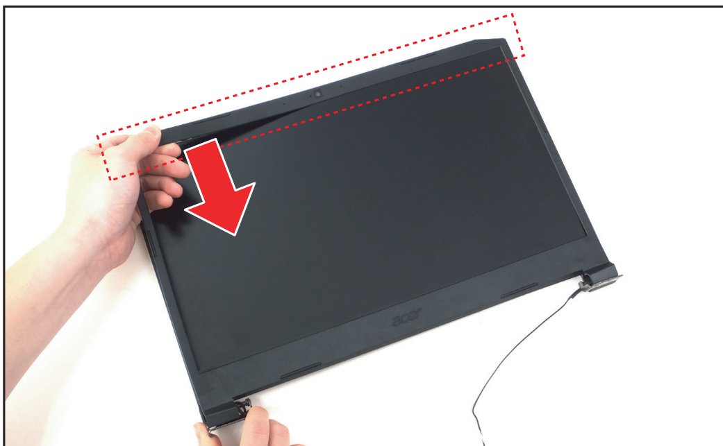
Figure 1-38. Retirer l'encadrement LCD (3 sur 3)
