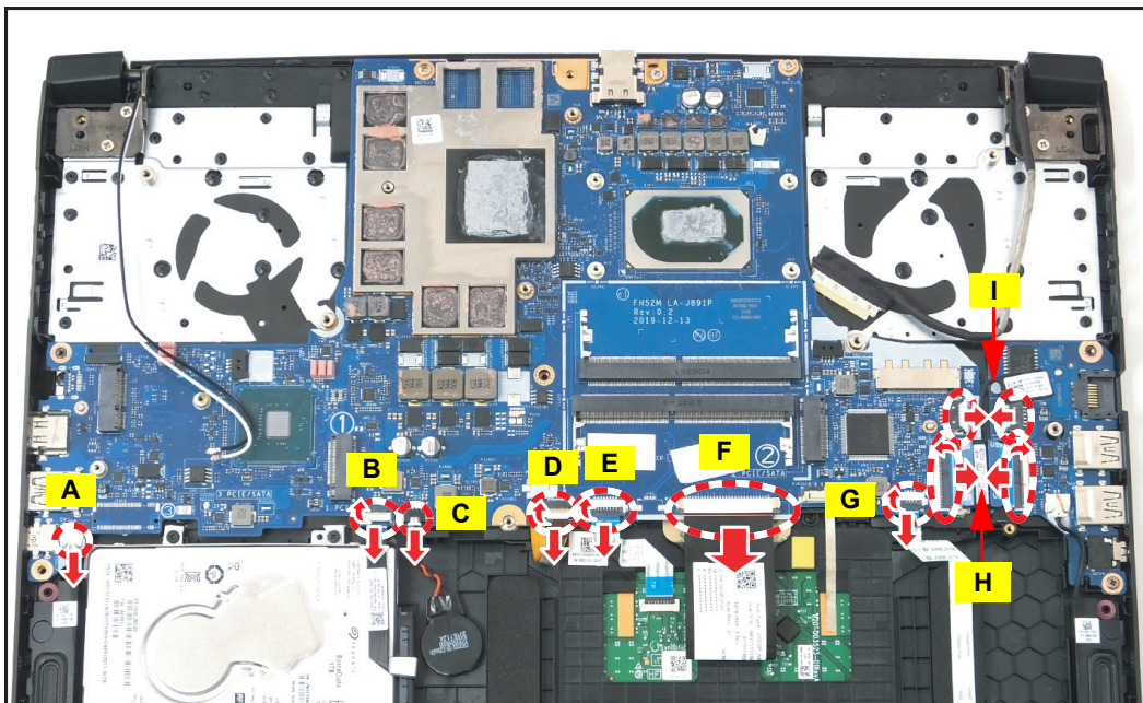
Figure 1-26. Débrancher les câbles
