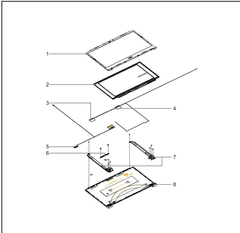
Figure 1-3. Vue éclatée de l'assemblage LCD
