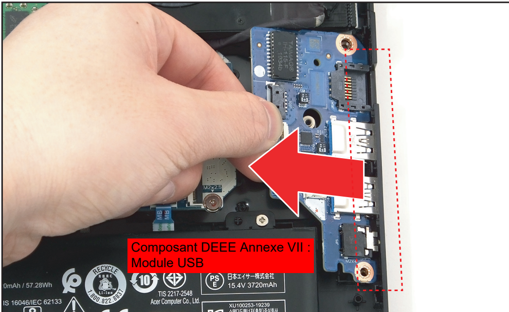
Figure 1-19. Retirer la carte USB
