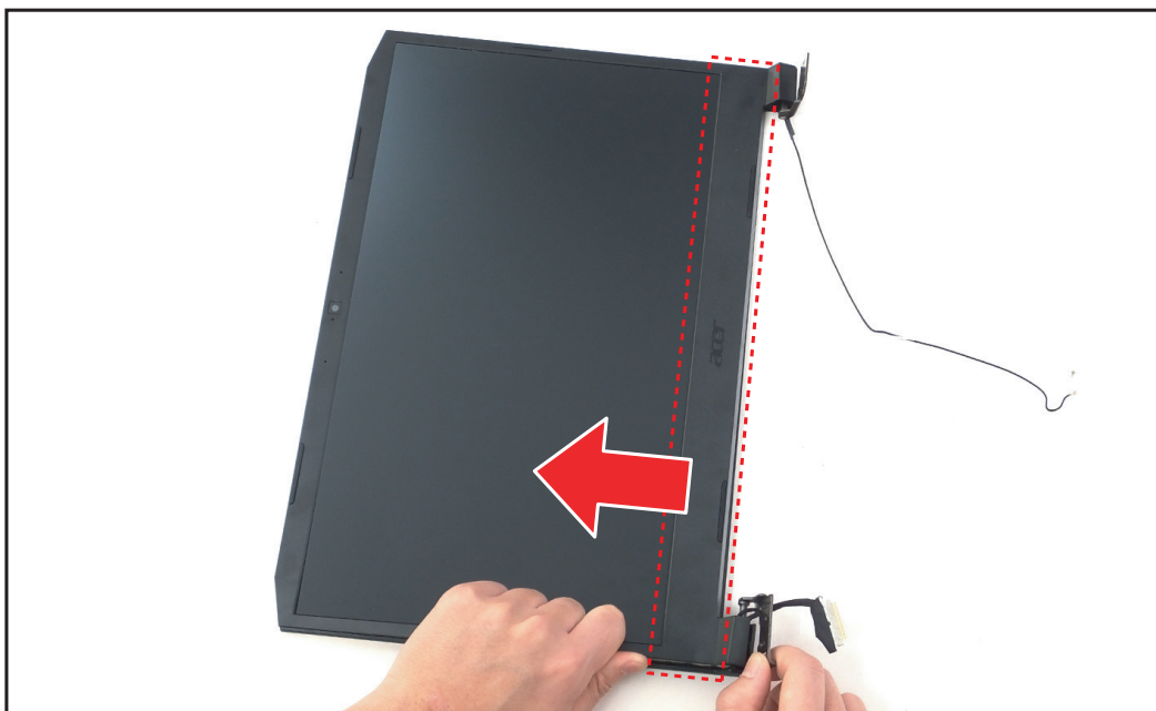
Figure 1-37. Retirer l'encadrement LCD (2 sur 3)
