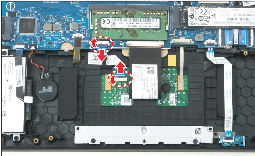
Figure 1-32. Retirer le câble plat et souple du pavé tactile
