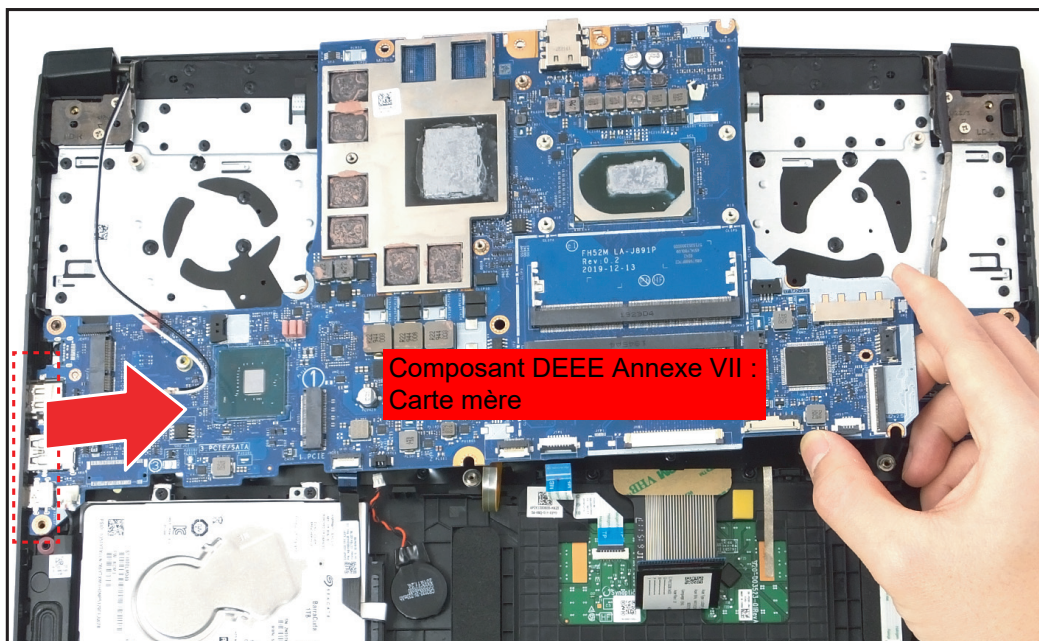
Figure 1-28. Retirer la carte mère
